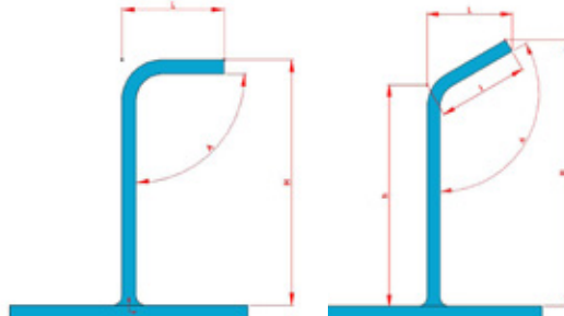
TACOS CURVOS A 90° O 120°
