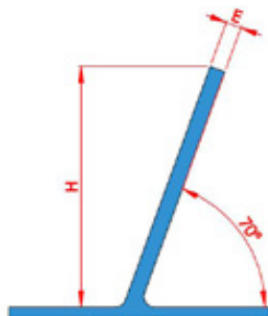
TACOS INCLINADOS A 70°C
